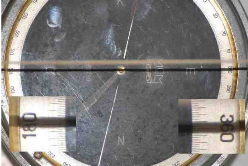
3.9. kép: Felfüggesztő kampók hibájának mérése
