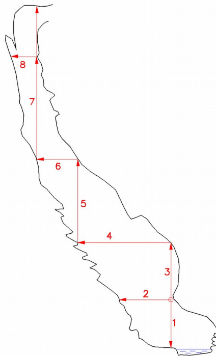
7. Ábra: Lépcsőzetes mérés poligon ponttól.
